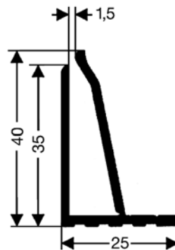
Fensteranschlussprofil
