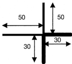
Eckprofil KI 10
