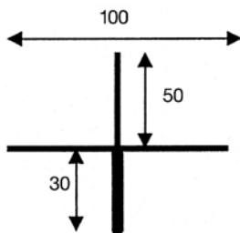
Linsenprofil KI 11 WD: Sichtschenkel: 4 mm Montageschenkel: 2 mm
